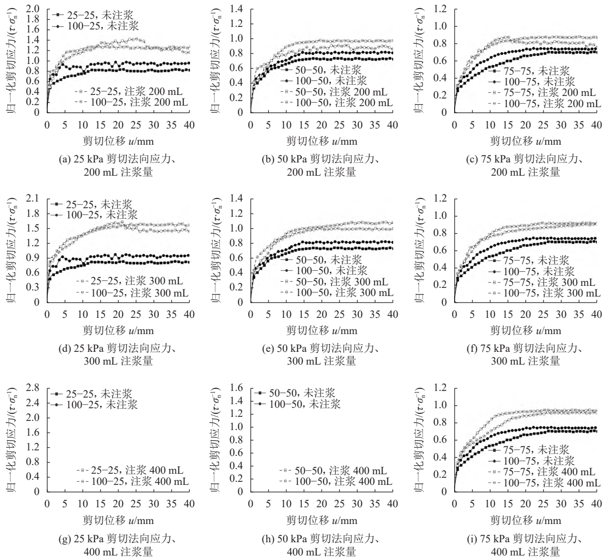
图 2 加、卸荷接触面归一化剪切应力-位移曲线
