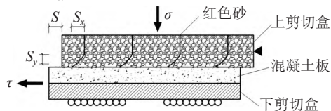
图1 剪切影响范围标志原理图
