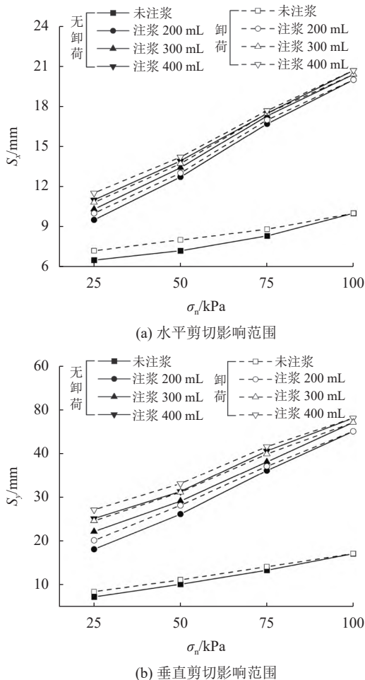
图 4 剪切影响范围随剪切法向应力变化曲线
